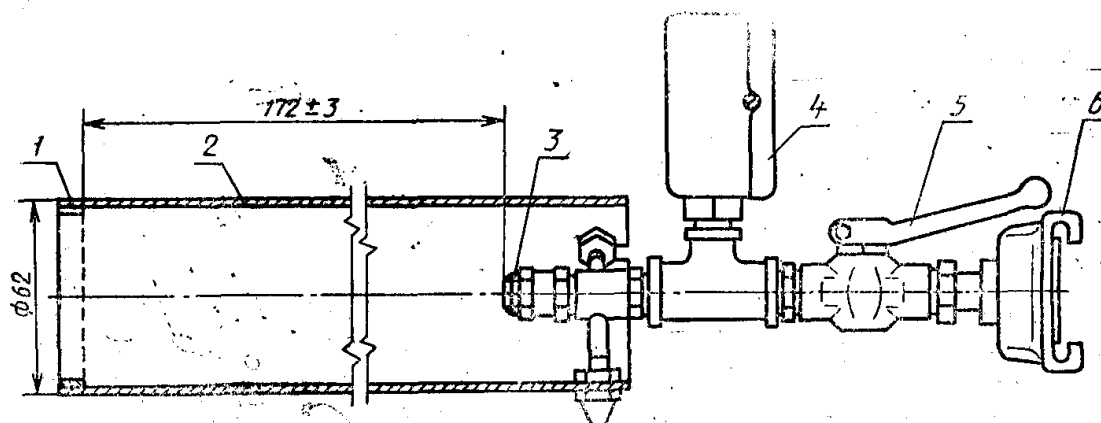
1—сетка; 2— корпус; 3—распылитель; 4 — манометр; 5—кран; 6—головка шторная ГМ-50 Черт. 6
