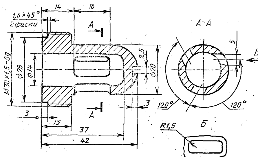
1 — корпус; 2 — пакет сеток; 3 — распылитель Черт. 2
