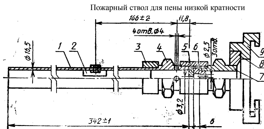
1 — труба; 2 — успокоитель; 3 — муфта; 4, 7 — штуцер; 5 — распылитель; 6. — смеситель; 8 — переходник; 9 — головка напорная ГМ-50 Черт. 3
