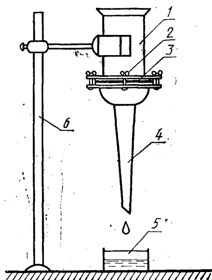
1 — цилиндр; 2 — винт; 3 — фильтр; 4 — сток; 5 — чашка; 6 — штатив Черт. 7
