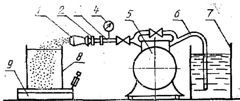
Схема установки для определения кратности и устойчивости пены
