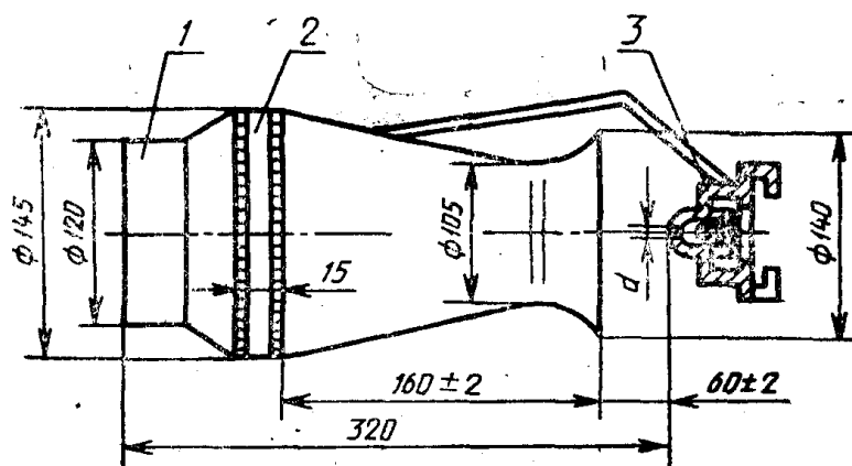
Генератор пены средней кратности ГПС-100
