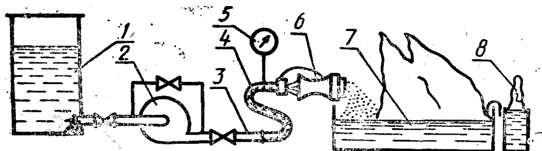
Схема установки для тушения пеной средней кратности
