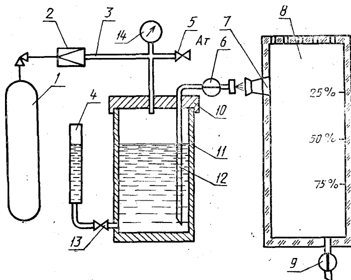
1—баллон для сжатого воздуха; 2—редуктор; 3—трубопровод; 4—мерная трубка; 5, 13 — клапан; 6, 9 — кран; 7 — генератор пены; 5—емкость; 10 — крышка; 11—сосуд; 12 — сифонная трубка; 14 — манометр
